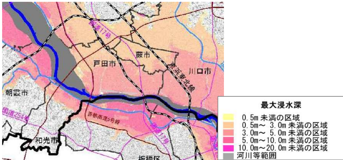
図 1-3-5 荒川氾濫時の浸水想定区域図（想定最大規模）
