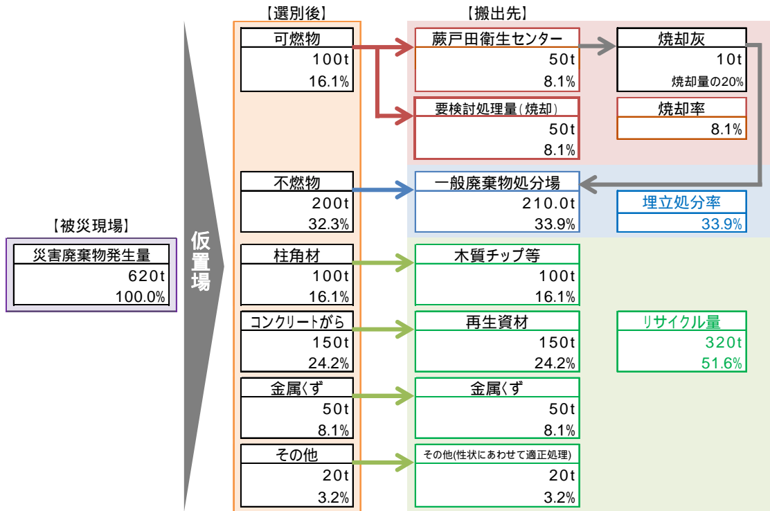
図2-1-5 基本の処理フロー
