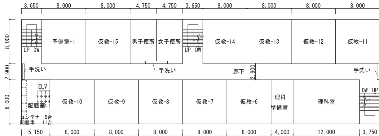
仮設校舎 (案) 3階平面図
